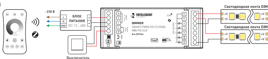
Рис. 1. Схемы подключения диммера SMART-PWM-105-72-RGB-MIX-PD-SUF
