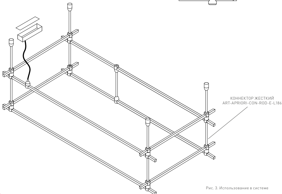
Рис. 2. Установка коннектора на шинопровод
