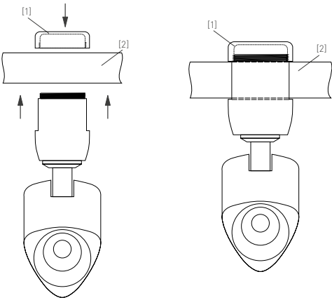
Рис. 2. Установка светильника
