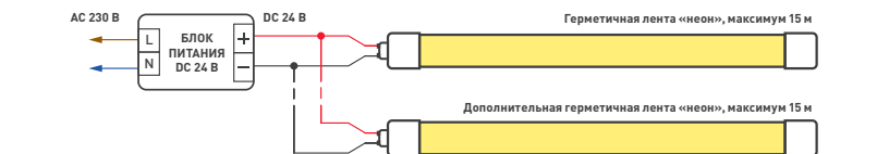
Схема 1. Подключение нескольких герметичных лент «неон» с одной стороны
